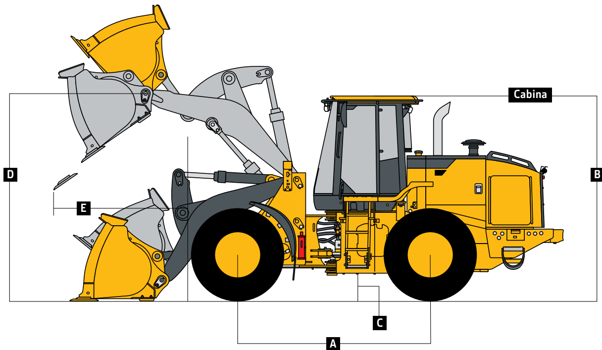
CARGADORES 724 P-TIER CON BARRA Z/ELEVACIÓN ALTA
